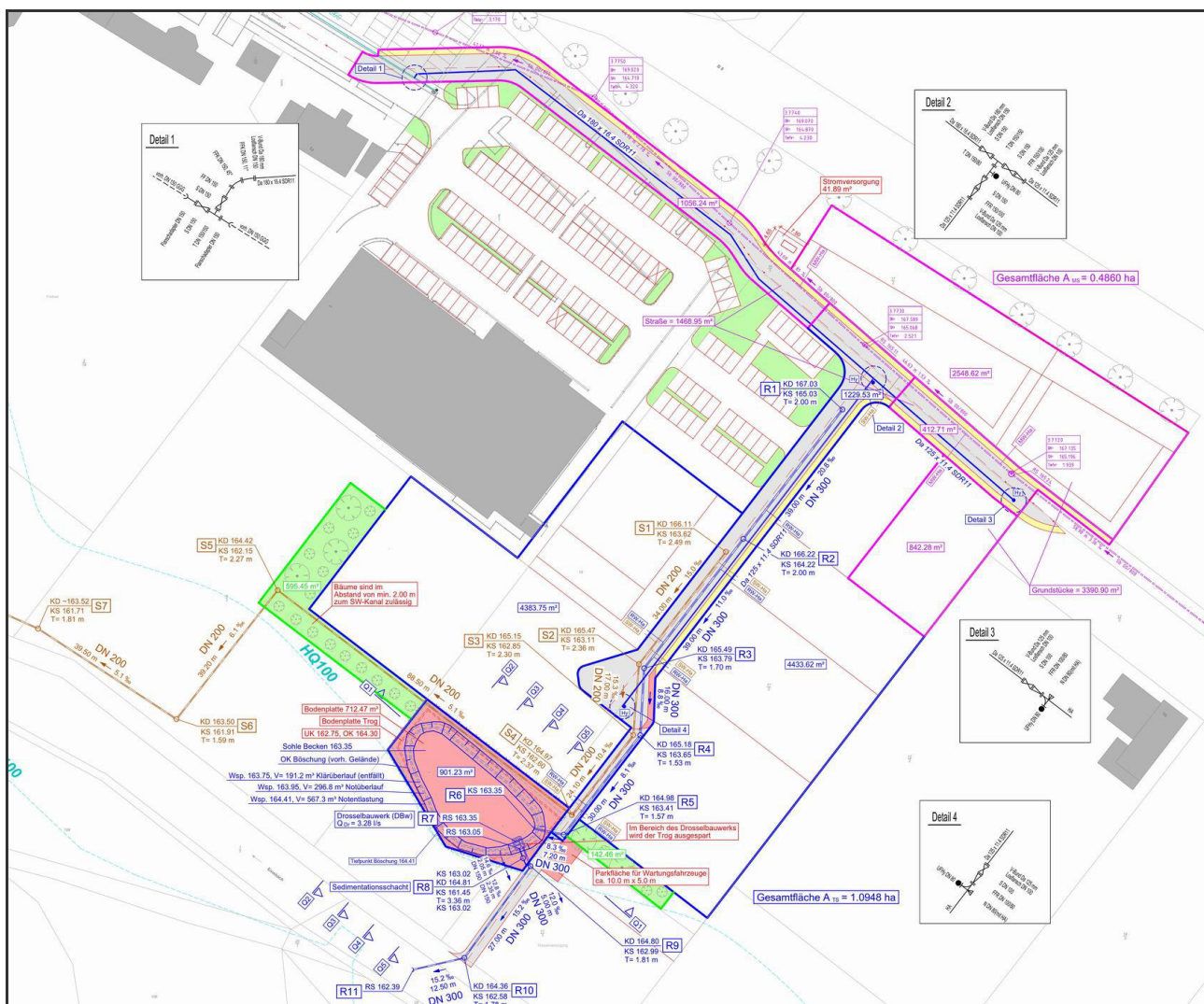
Erschließungsplanung (unmaßstäblich, Werner Hartwig GmbH August 2024)
